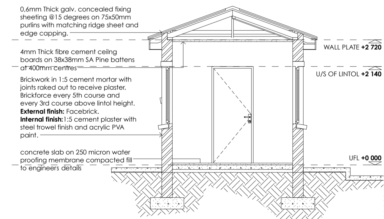
Section D-D 1:50
